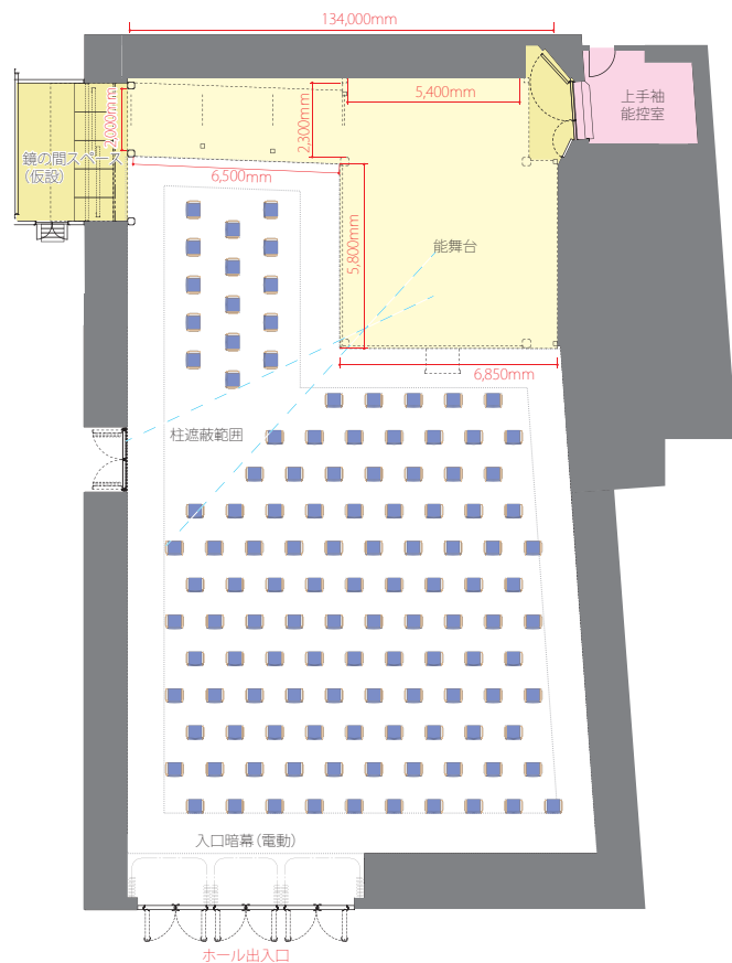
能舞台レイアウト(120席)
